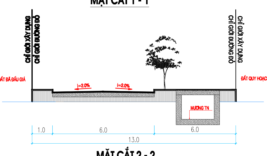
MẶT CẮT 2 - 2
