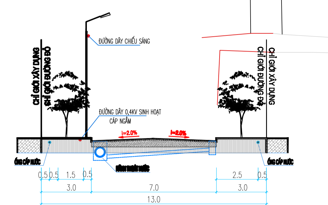
MẶT CẮT 1 - 1
